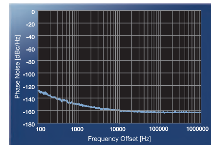
400MHz HRDDS Unit
